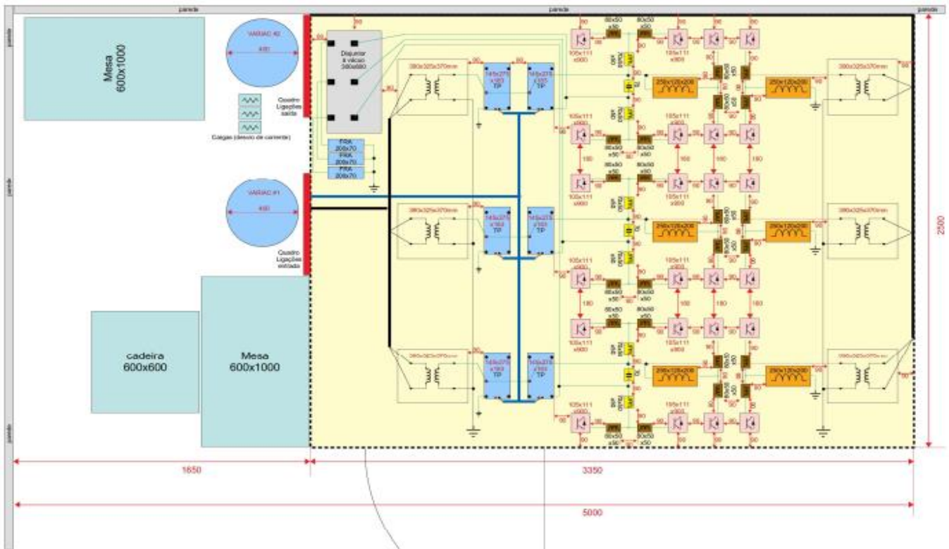
Planta baixa do Laboratório de Média Tensão
