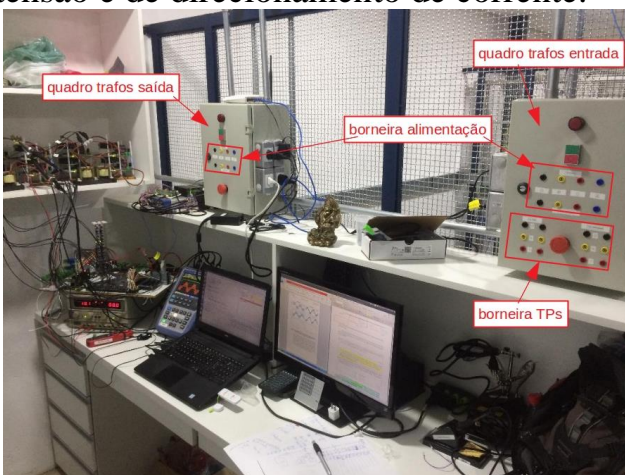
Sala de Controle e Área de Teste dos Equipamentos
